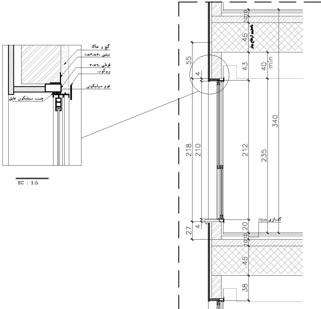
برش عمودی از پنجره
