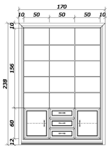
E-13-2 Sc:1/25
